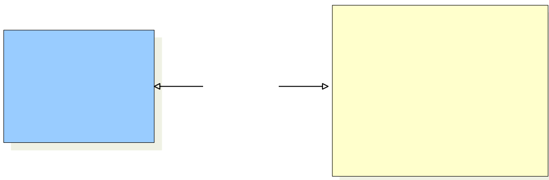
Abbildung 31: Systemumgebung Mitversicherungsportal
